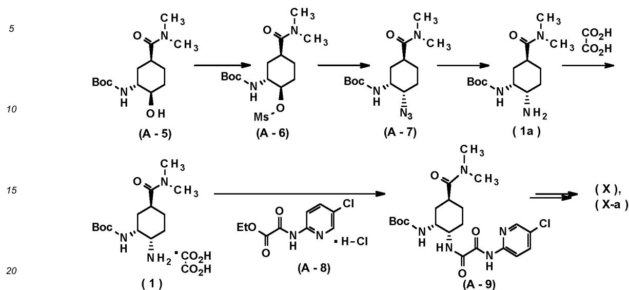
[Scheme A]
