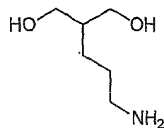
2-(1-Aminopropyl)-1,3-propanediol
