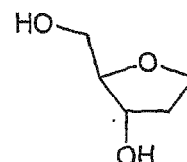
1,2-Dideoxyribose
