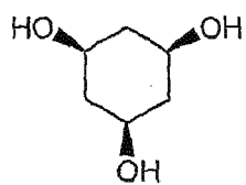
cis-1,3,5-Cyclohexanetriol
