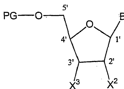
LCM-I
