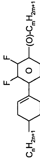
CYLI-n-m
