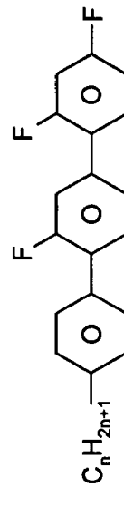
LYLI-n-m
