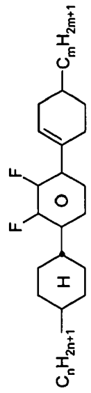
CPQIY-n-Om
