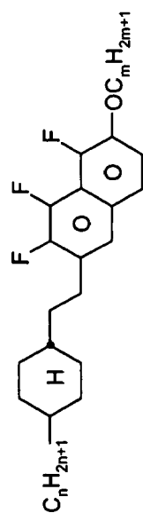
CENap-n-Om
