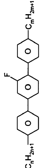
LY-n-(O)m
