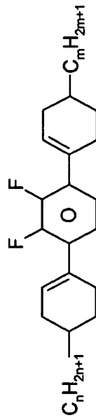
CLY-n-(O)m
