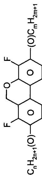
DFDBC-n(O)-(O)m
