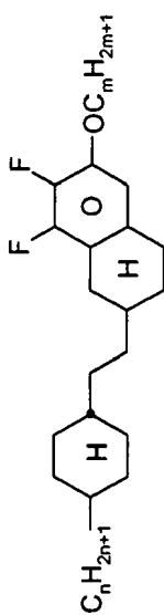
CENap-n-Om
