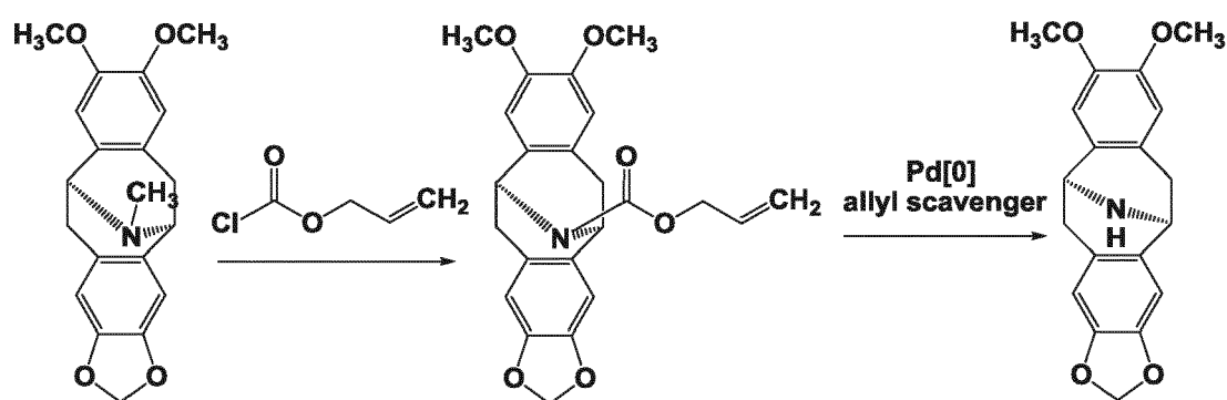
Scheme 26: (+)-Eschscholtzidine
