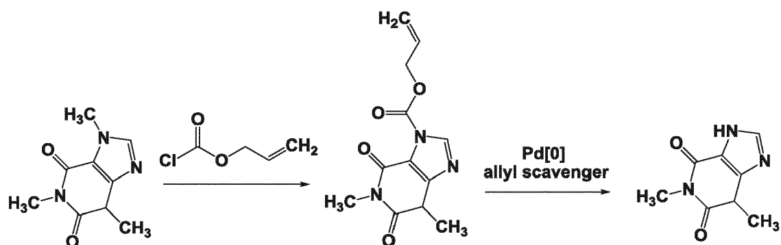
Scheme 26: (+)-Eschscholtzidine
