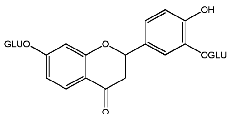
Butrin (m/z = 596)
