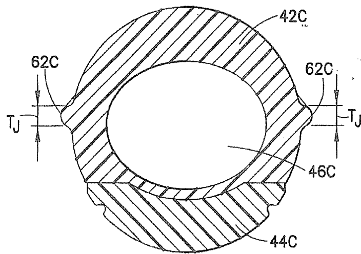
FIG. 35C1
