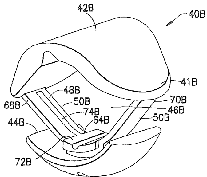
FIG. 35N
