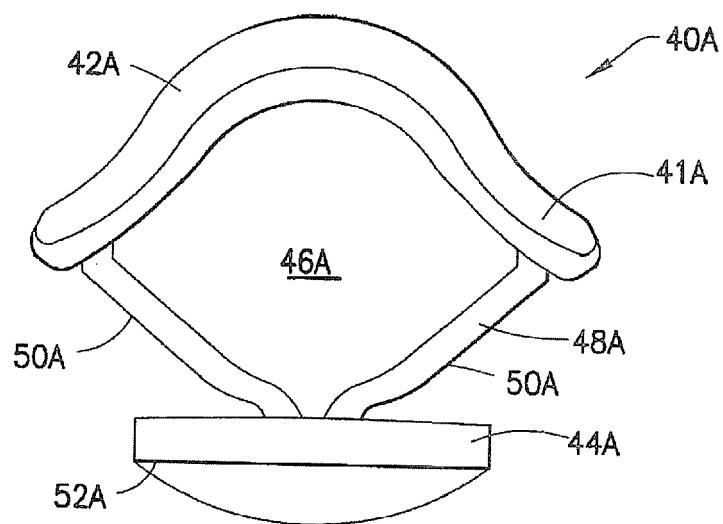
FIG. 35G
