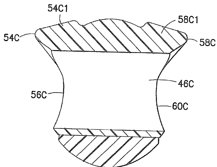
FIG.35D
