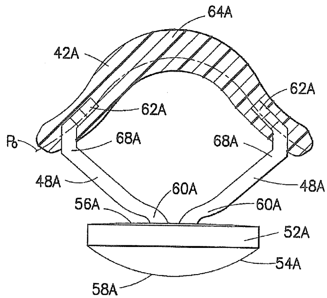
FIG.35H
