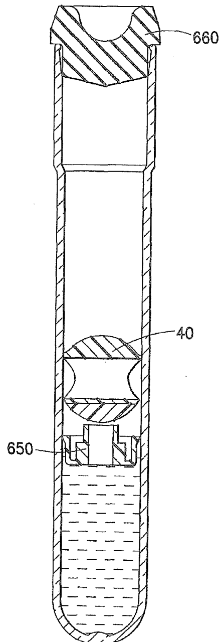
FIG.64
