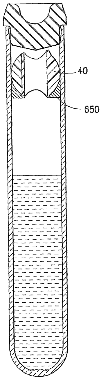
FIG.67
