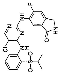
6-(4-(2-(isopropylsulfonyl)phenylamino)-5-chloropyrimidin-2-ylamino)-5-fluoroisoindolin-1-one
