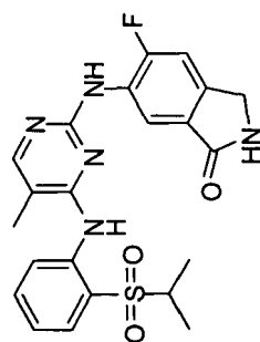
6-(4-(2-(isopropylsulfonyl)phenylamino)-5-chloropyrimidin-2-ylamino)-5-fluoroisoindolin-1-one
