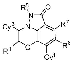
(IIb)
