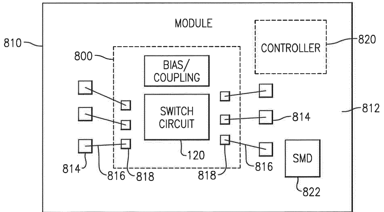
FIG.30A
