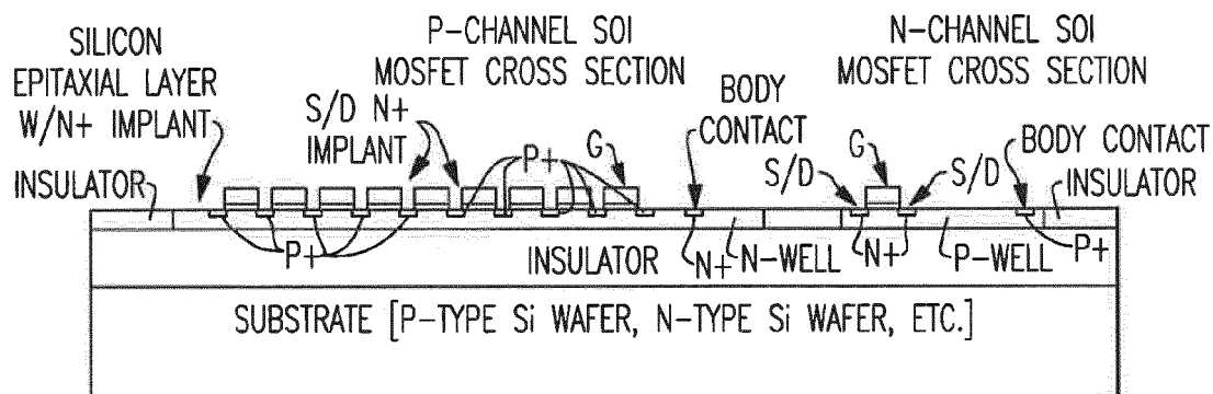
FIG. 28B
