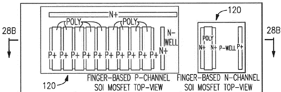
FIG. 28A
