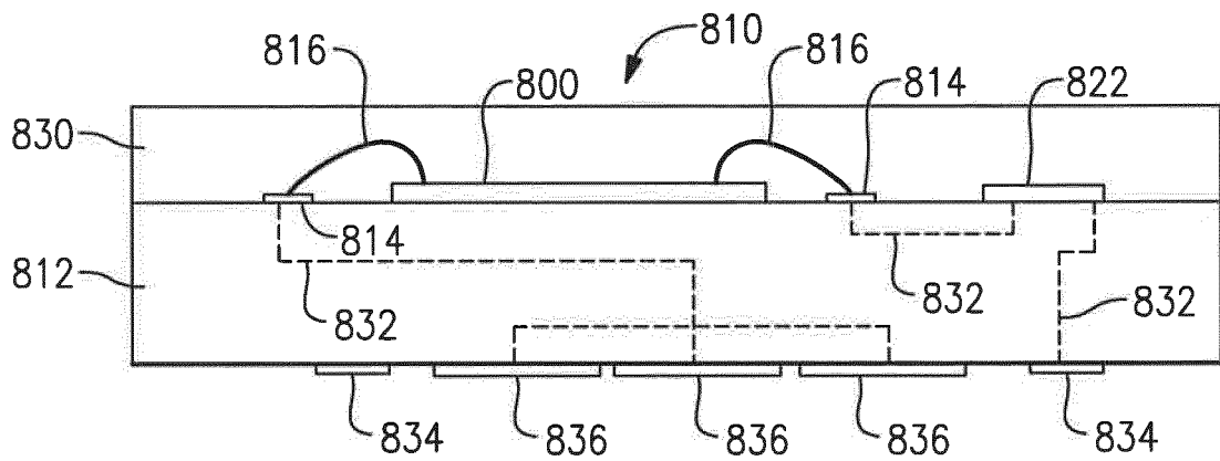
FIG.30B
