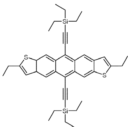
Compound (D)
