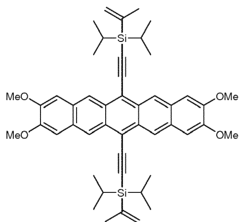
Compound (D)
