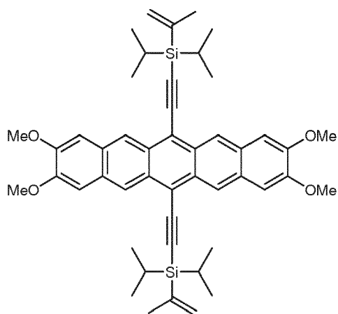
Compound (D)
