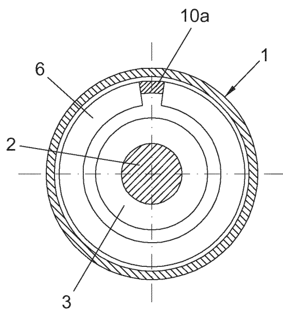
FIG. 6 SEC. C-D
