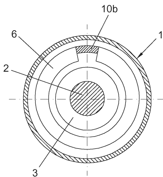
FIG. 5 SEC. A-B
