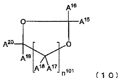
[Chem. 23]
