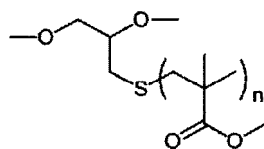
PMMA-OH2 (Mn=10,000)
