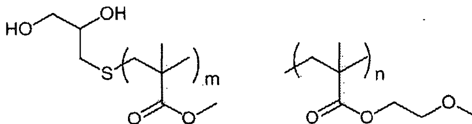
PMMA-OH2 (Mn=10,000)
