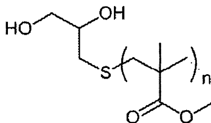
PMMA-OH2 (Mn=10,000)
