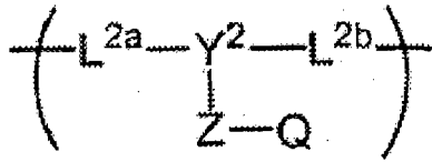
Formule (B)
