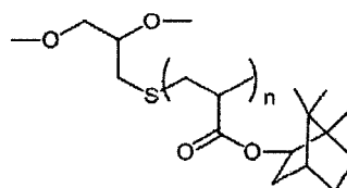
PIBOA-OH2 (Mn=8,000)
