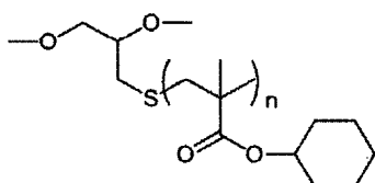
PCyHMA-OH2 (Mn=6,000)
