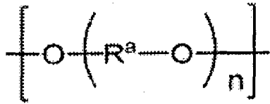
Formule (C)
