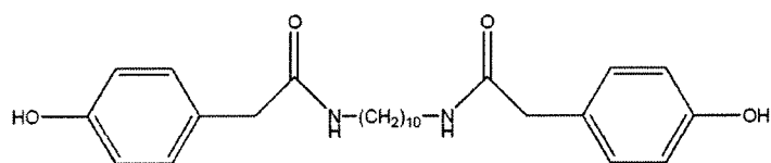
Formel (IA);
