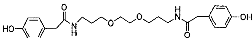
Formule (IB).
