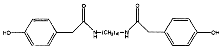
Formule (IA)
