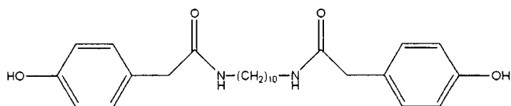
Formula (IA);
