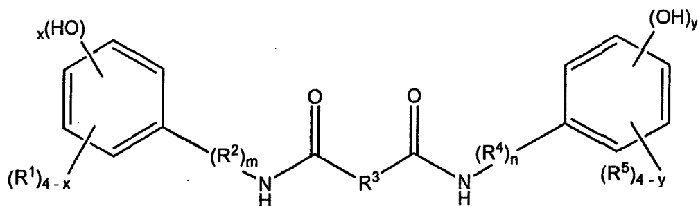
Formule (II)
