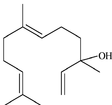
nerolidol (CAS #7212-44-4)
