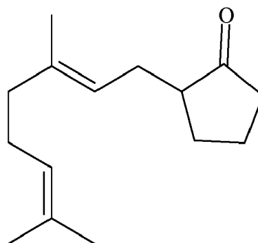
apritone (CAS #68133-79-9)
