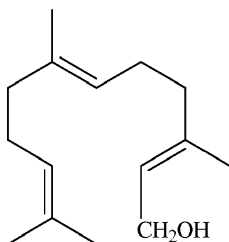
farnesol (CAS #4602-84-0)
