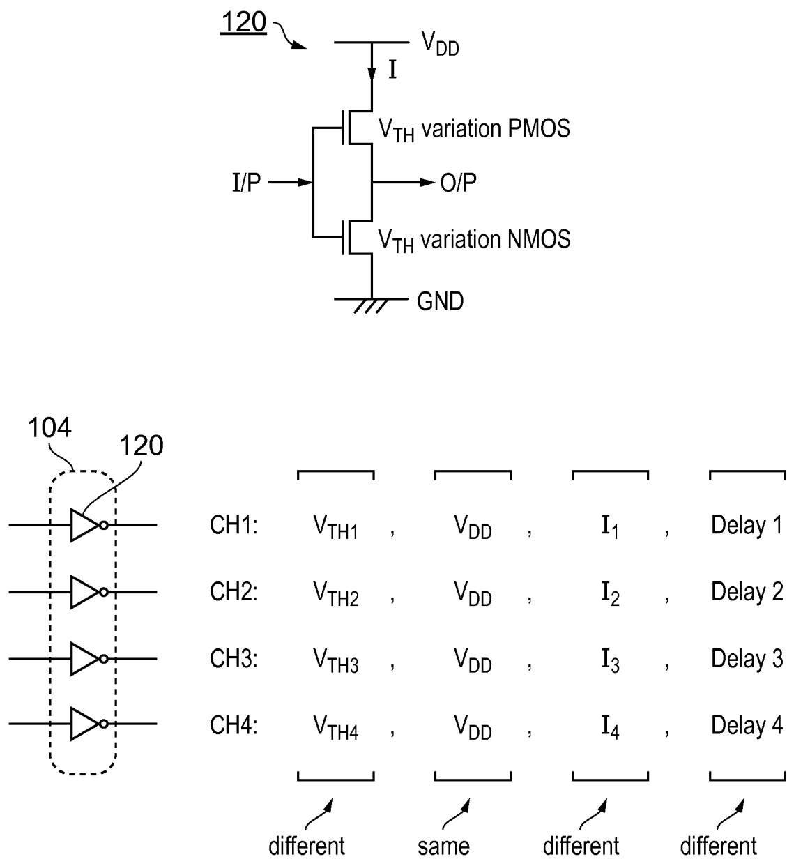
FIG. 8A
