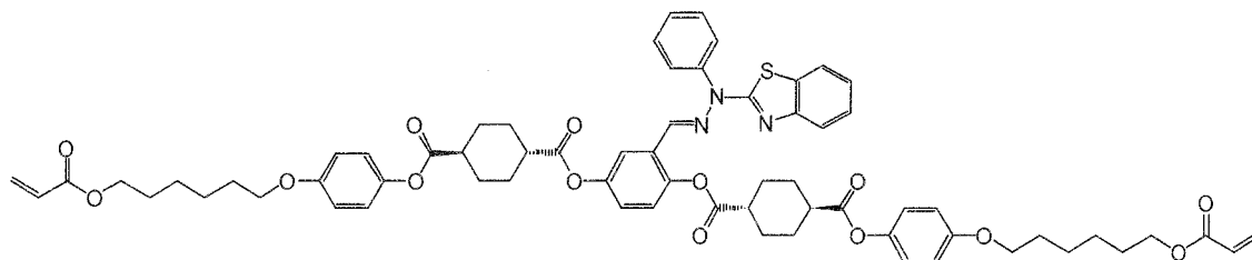
Compound 1r
