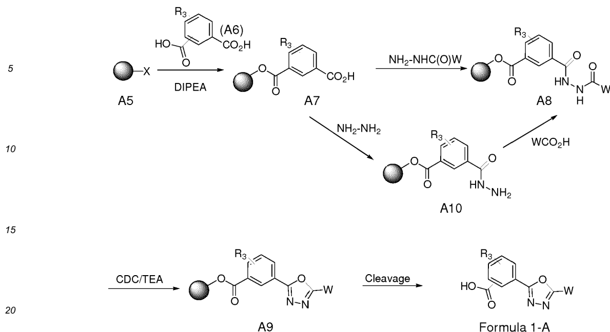
Scheme A3
