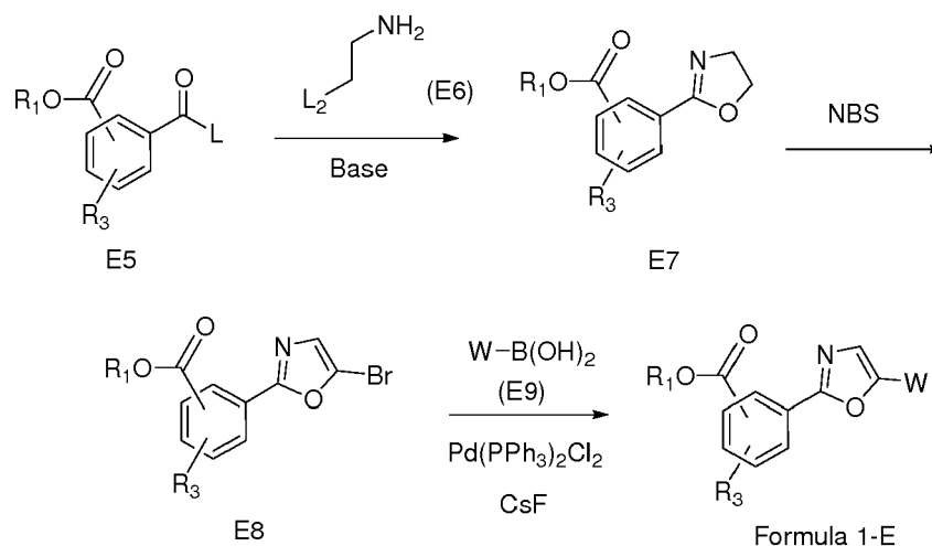
Scheme E2
