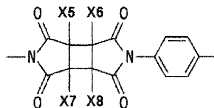
chemische Formel 10
