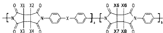
chemische Formel 11
