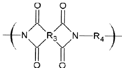
Formule chimique 5
