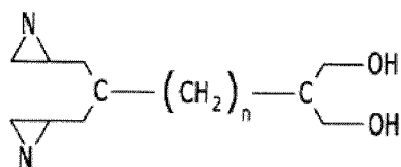
Formule chimique 1-1
