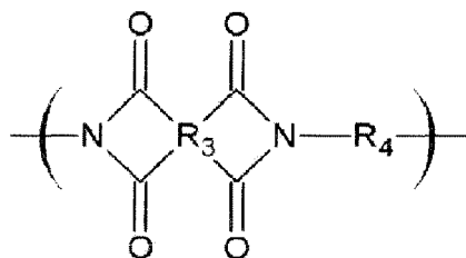
chemische Formel 5
