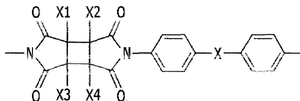
chemische Formel 9
