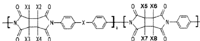
Formule chimique 11
