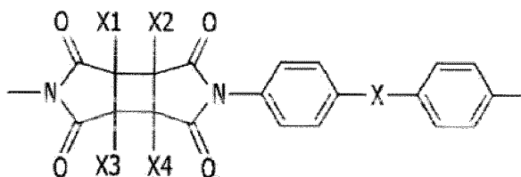
Formule chimique 9
