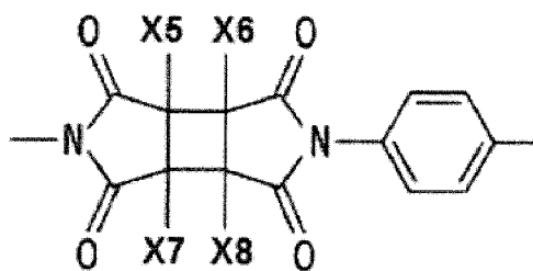
Formule chimique 10
