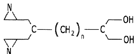
chemische Formel 1-1
