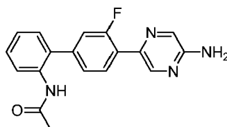
N -[4'-(5-Aminopyrazin-2-yl)-3'-fluorobiphenyl-2-yl]acetamide
