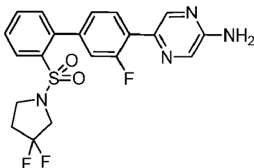
5-{2'-[(3,3-Difluoropyrrolidin-1-yl)sulfonyl]-3-fluorobiphenyl-4-yl}pyrazin-2-amine
