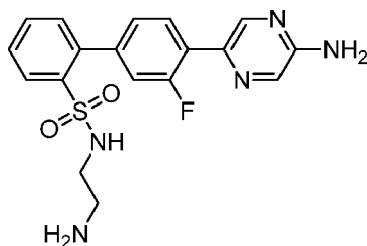
N -(2-Aminoethyl)-4'-(5-aminopyrazin-2-yl)-3'-fluorobiphenyl-2-sulfonamide
