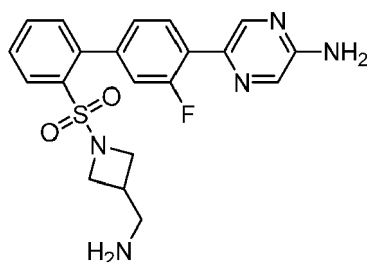
5-(2'-[3-(Aminomethyl)azetidin-1-yl]sulfonyl)-3-fluorobiphenyl-4-ylpyrazin-2-amine
