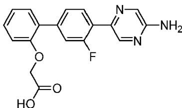
{4'-(5-Aminopyrazin-2-yl)-3-fluorobiphenyl-2-yl[oxy]}acetic acid
