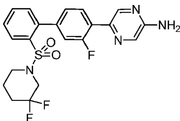
5-{2'-[(3,3-Difluoropiperidin-1-yl)sulfonyl]-3-fluorobiphenyl-4-yl}pyrazin-2-amine
