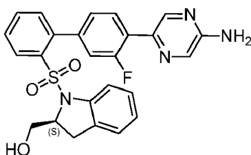
(S)-(1-([4'-(5-Aminopyrazin-2-yl)-3'-fluorobiphenyl-2-yl]sulfonyl)-2,3-dihydro-1H-indol-2-yl)-methanol
