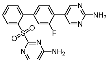
5-{2'-[(4-Aminopyrimidin-2-yl)sulfonyl]-3-fluorobiphenyl-4-yl}pyrimidin-2-amine
