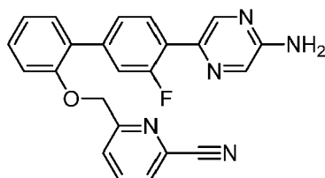
6-([4'-(5-Aminopyrazin-2-yl)-3'-fluorobiphenyl-2-yl]oxy)methylpyridine-2-carbonitrile
