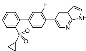
5-[2'-(Cyclopropylsulfonyl)-3-fluorobiphenyl-4-yl]-1H-pyrrolo[2,3-b]pyridine
