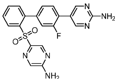
5-{2'-[(5-Aminopyrazin-2-yl)sulfonyl]-3-fluorobiphenyl-4-yl}pyrimidin-2-amine
