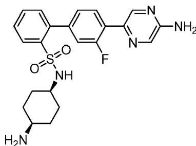
cis -N-(4-Aminocyclohexyl)-4'-(5-aminopyrazin-2-yl)-3'-fluorobiphenyl-2-sulfonamide
