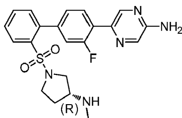
(R)-5-(3-Fluoro-2'-[3-(methylamino)pyrrolidin-1-yl]sulfonyl)biphenyl-4-ylpyrazin-2-amine
