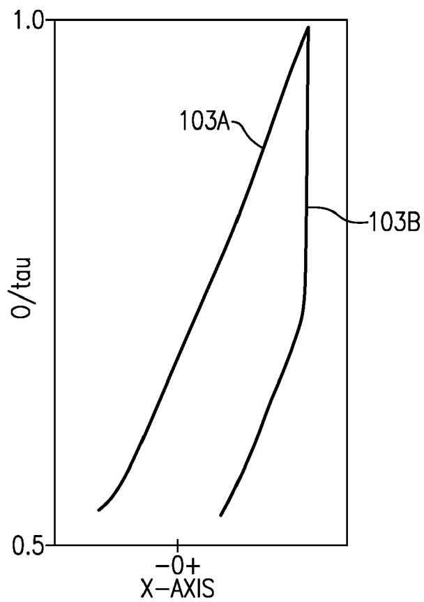
FIG. 6F
