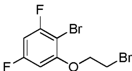
2-Bromo-1-(2-bromoethoxy)-3,5-difluorobenzene
