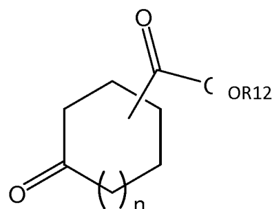
Formule VII
