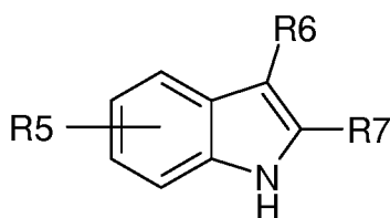
Formel VIII
