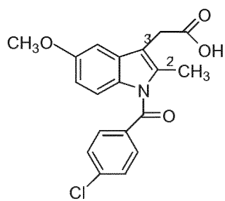
Indometacin
