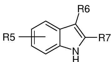
Formule VIII
