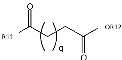
Formule VI
