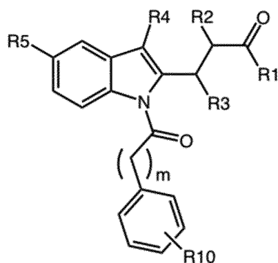
Formule II,
