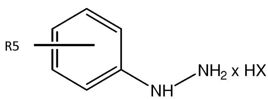
Formule V
