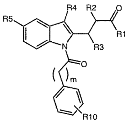
Formule II,
