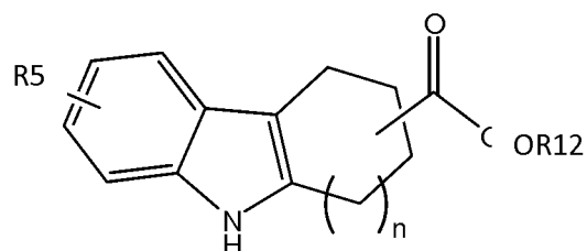
Formule IX
