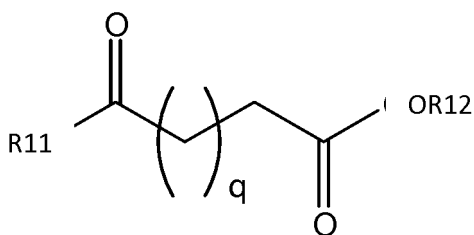
Formel VI
