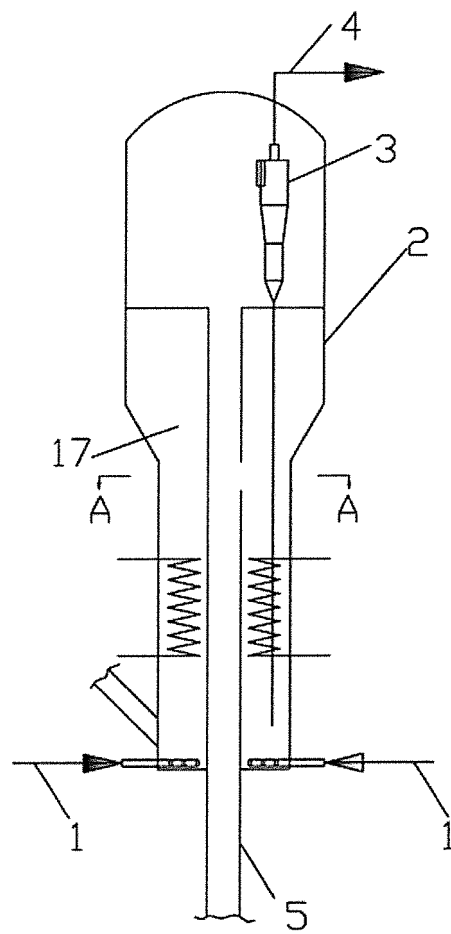
A-A section
