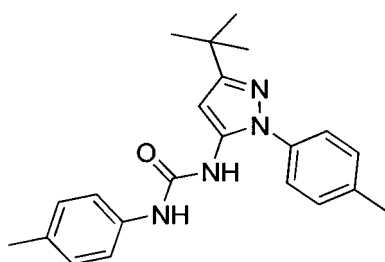
1-(3-tert-butyl-1-p-tolyl-1H-pyrazol-5-yl)-3-p-tolylurea
