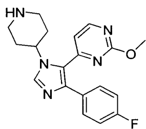
SB-242235
