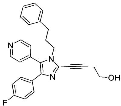
RWJ 67657
