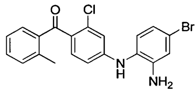
EO 1428
