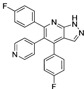
Org 48762-0
