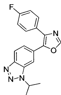
4-(4-fluorophenyl)-5-(1-isopropyl-1H-benzo[d][1,2,3]triazol-6-yl)oxazole
