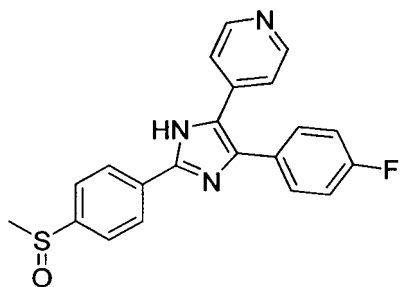
SB-203580
