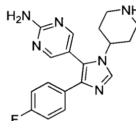
SB 220025
