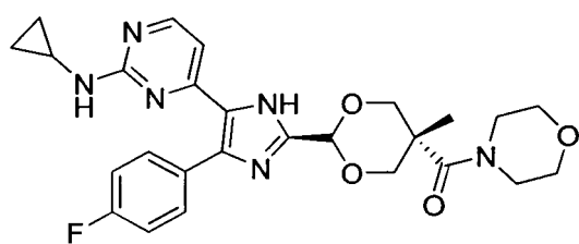
RPR-203494
