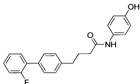
CMPD1
