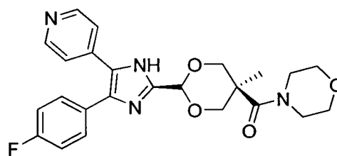
RPR-200765A
