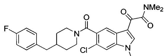
SX 011
