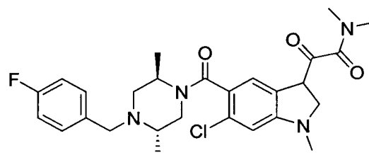
SCIO 469
