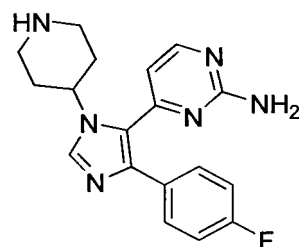
SB-200025
