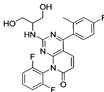
SCIO 469
