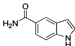
SD 282
