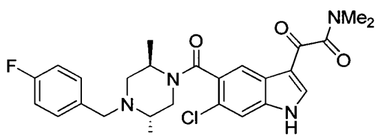
SD 282
