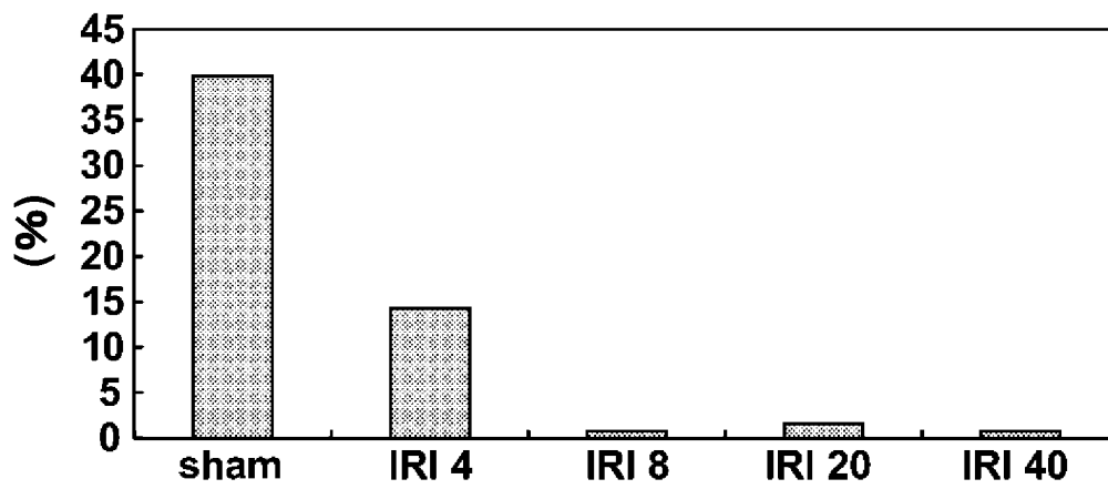
FIG. 4-A D-His/D-His+L-His
