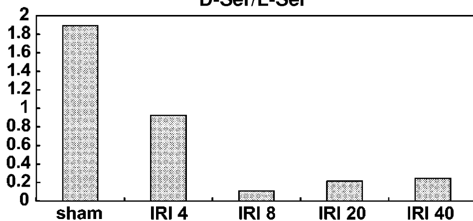
FIG. 3-C D-Ser/L-Ser
