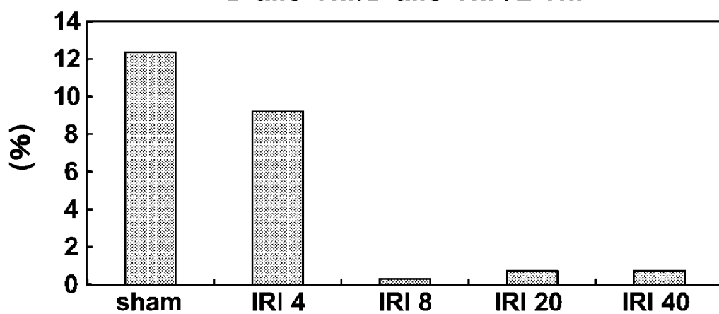
FIG. 4-E D-allo-Thr/D-allo-Thr+L-Thr
