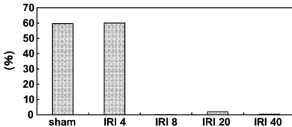
FIG. 4-J D-allo-Ile/D-allo-Ile+L-Ile
