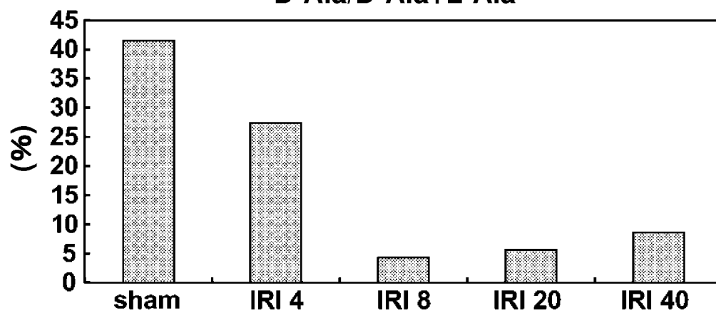
FIG. 4-G D-Ala/D-Ala+L-Ala
