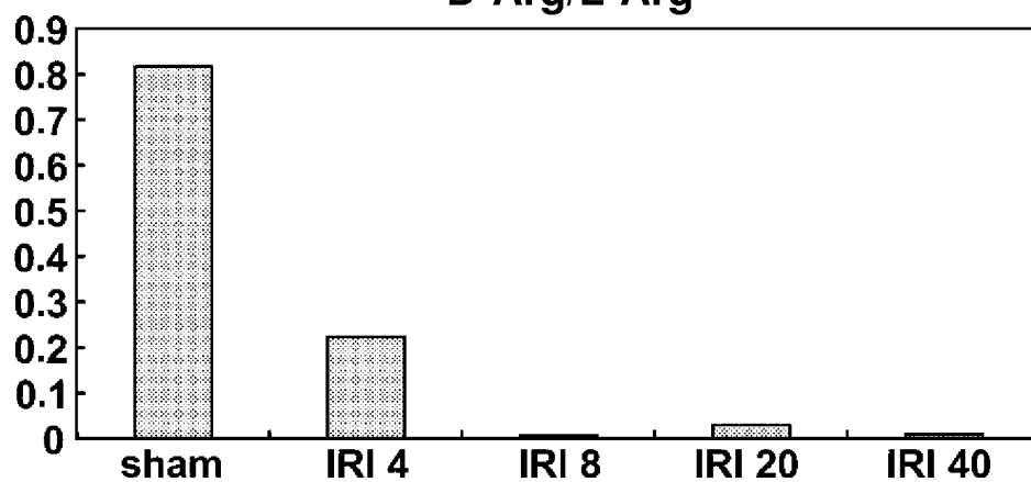
FIG. 3-D D-Arg/L-Arg
