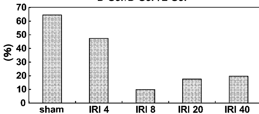
FIG. 4-C D-Ser/D-Ser+L-Ser
