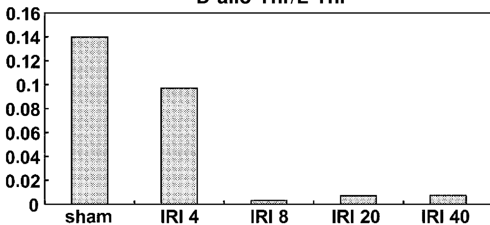
FIG. 3-E D-allo-Thr/L-Thr
