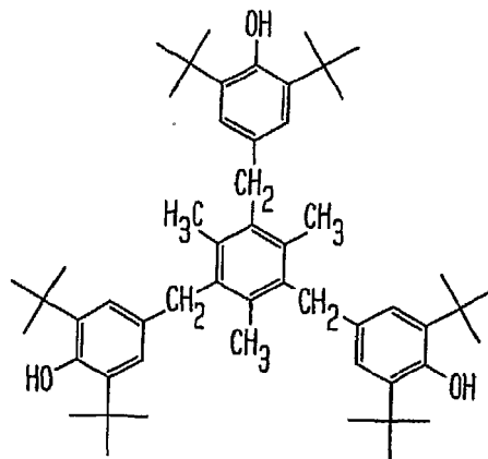
IRGANOX ® 1330
