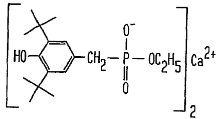
IRGANOX ® 1425
