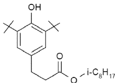
Ciba® Irganox® 1135;
