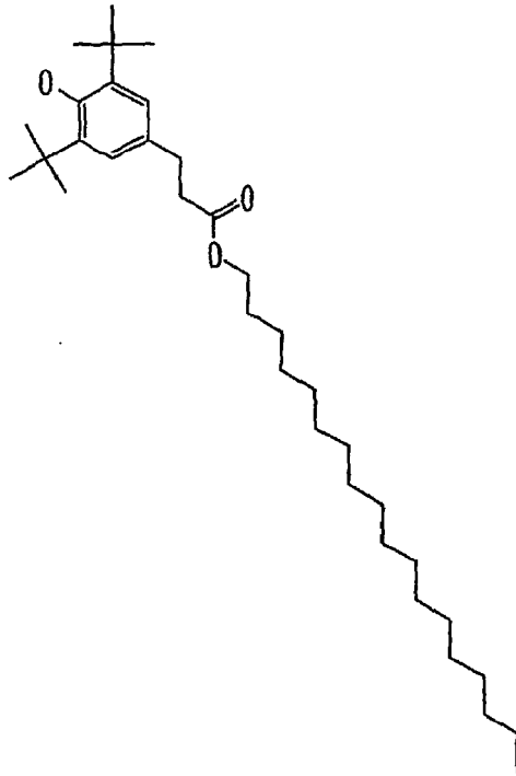
IRGANOX ® 1076
