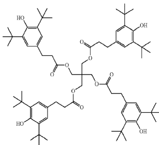
Ciba® Irganox® 1010;
