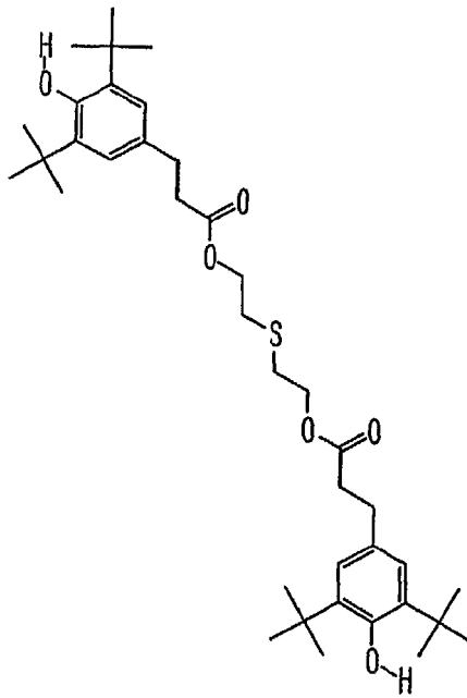
IRGANOX ® 1035
