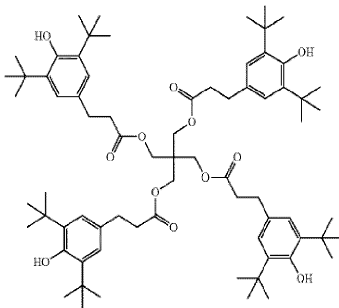
Ciba® Irganox® 1010.
