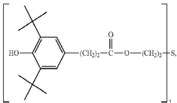
Ciba® Irganox® 1035;
