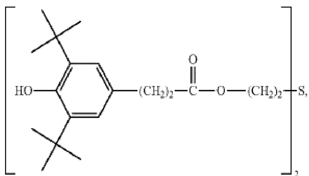
Ciba® Irganox® 1035;
