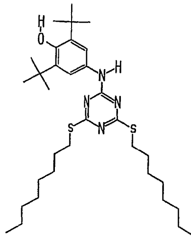
IRGANOX ® 565
