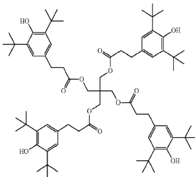
Ciba® Irganox® 1010;
