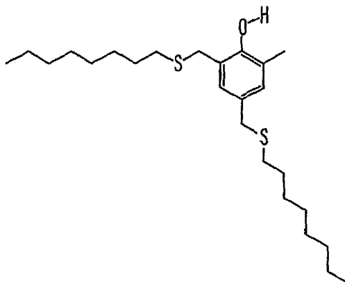
IRGANOX ® 1520
