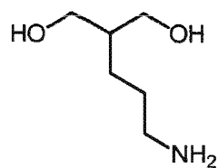
2-(1-Aminopropyl)-1,3-propanediol
