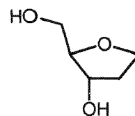
1,2-Dideoxyribose
