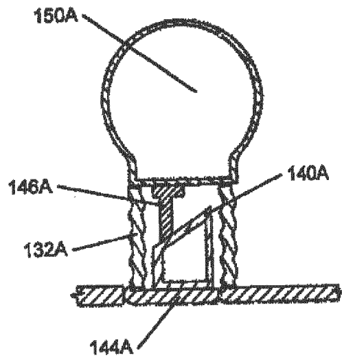
FIG. 2A1
