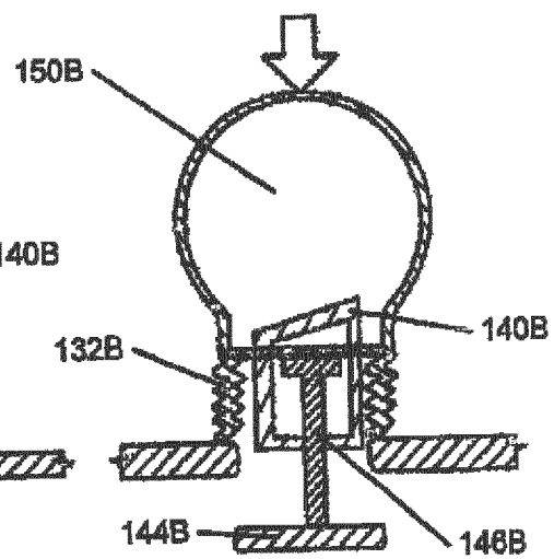
FIG. 2B2
