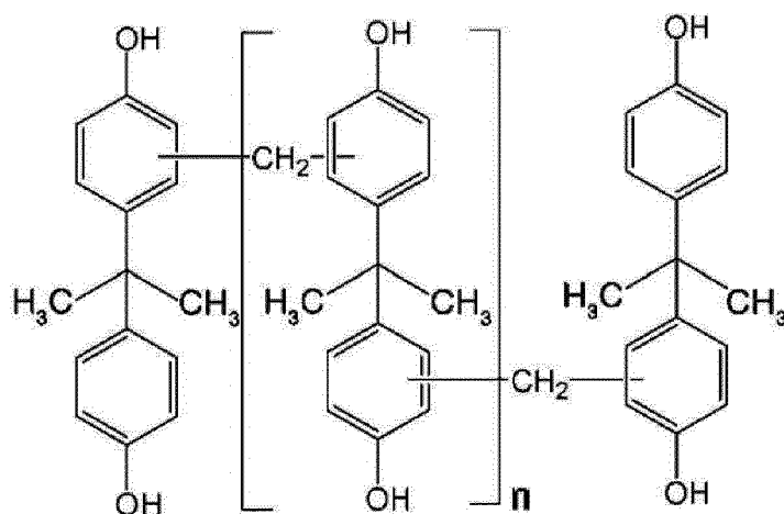
[Formula IA-4]
