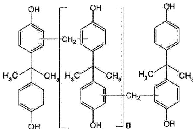
[Formula IA-4]
