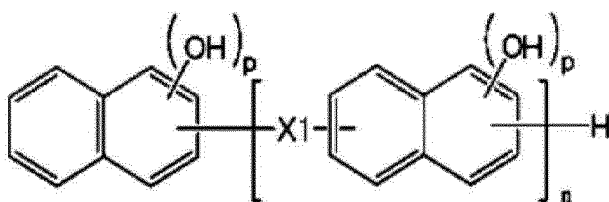
[Formula IA-4]
