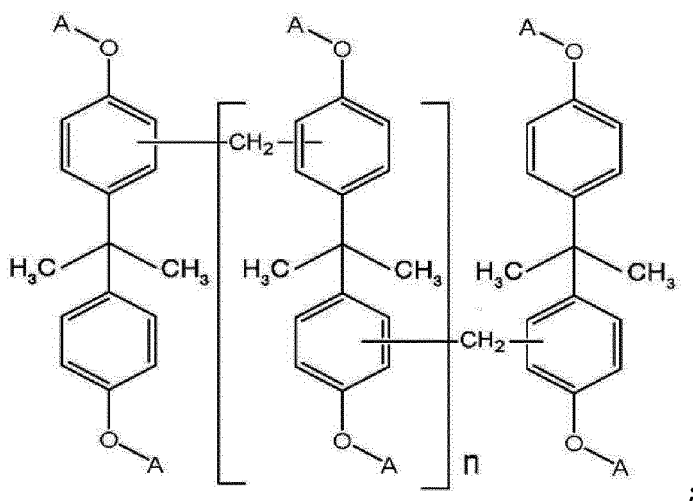
[Formula I-3]
