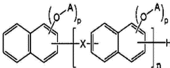
[Formula I-4]
