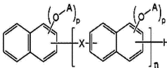
[Formula I-4]
