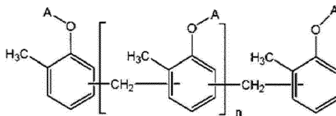
[Formula I-3]
