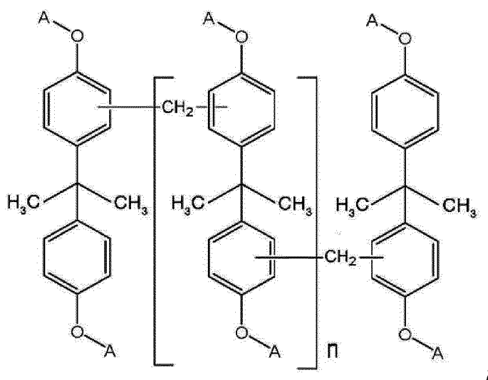
[Formula I-3]
