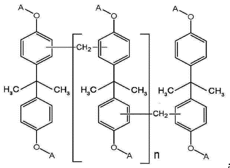
[Formula I-3]
