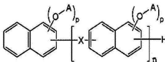
[Formula I-4]
