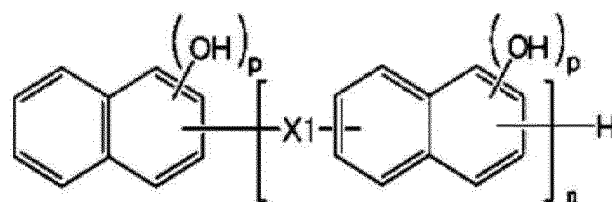
[Formula IA-4]
