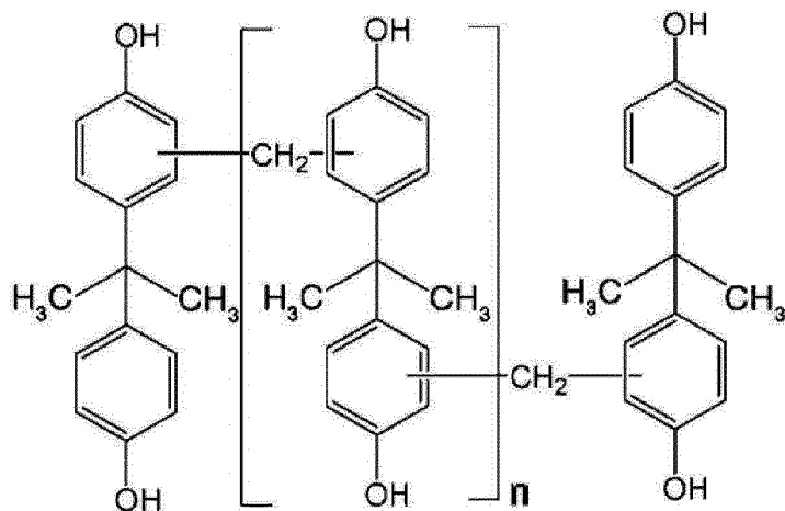
[Formula IA-4]
