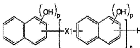
[Formula IA-4]
