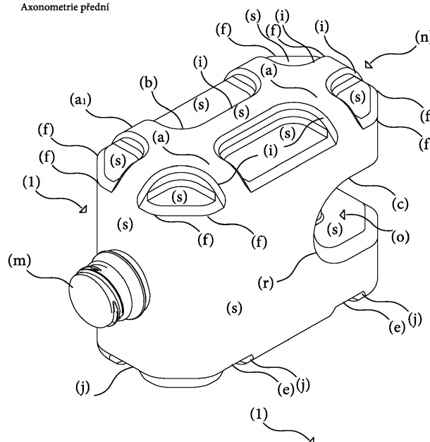
Axonometrie přední
