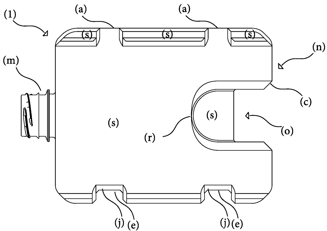
Pohled shora
