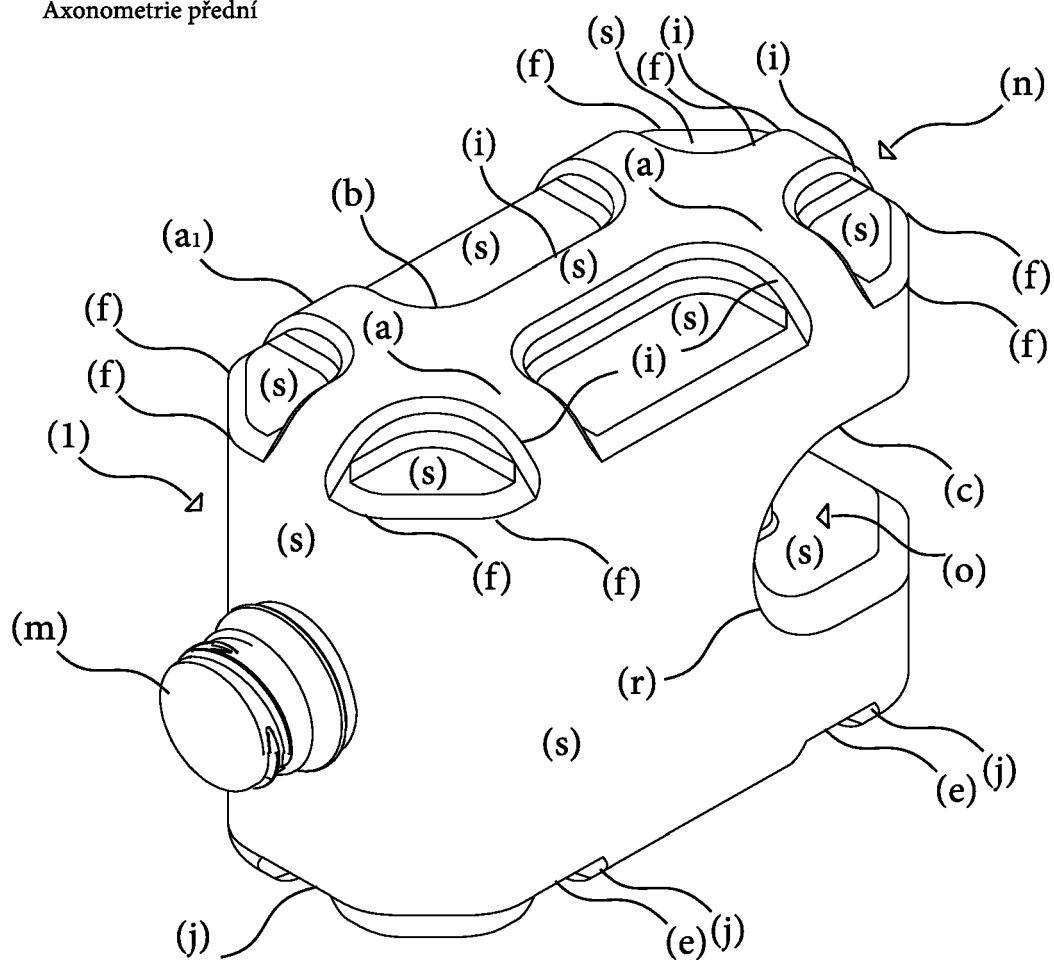
Pohled zespoda
