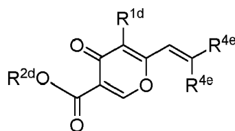
( XA3 )
