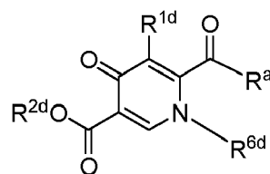
( XA4 )
