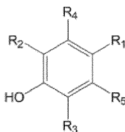
[Formule Chimique 1]
