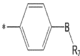
[Formule Chimique 3]
