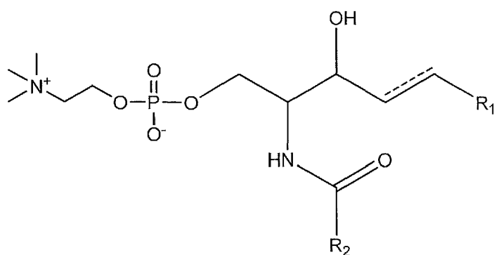
(IV)
