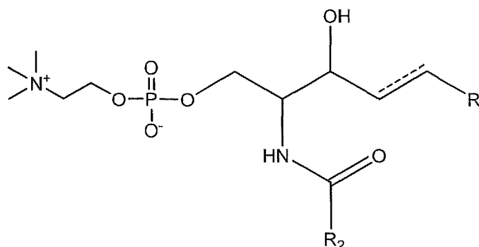
(IV)
