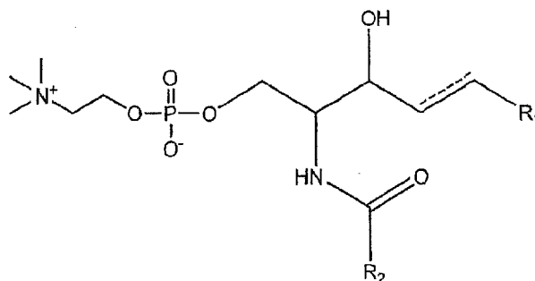
(IV)
