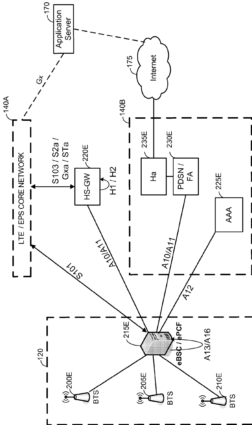
FIG. 2E eHRPD EXAMPLE
