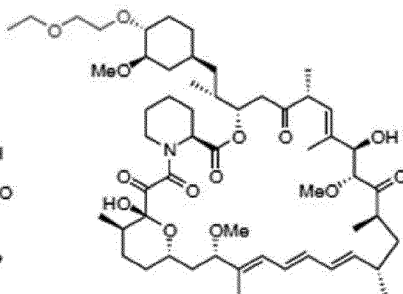
Umirolimus
