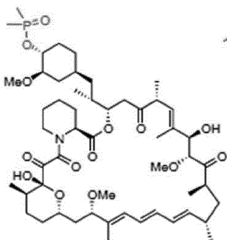
Ridaforolimus (MK-8669)
