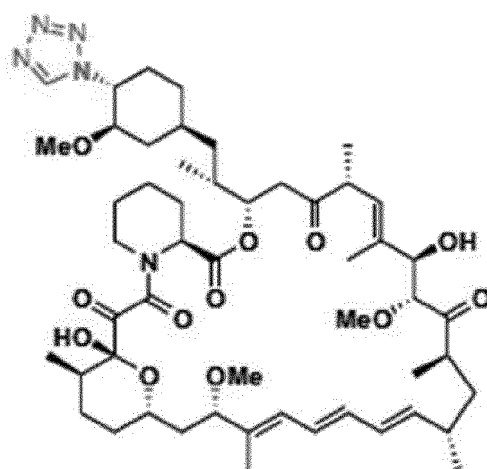
Zotarolimus (ABT-578)
