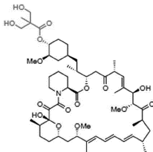
Temsirolimus (CCI-779)
