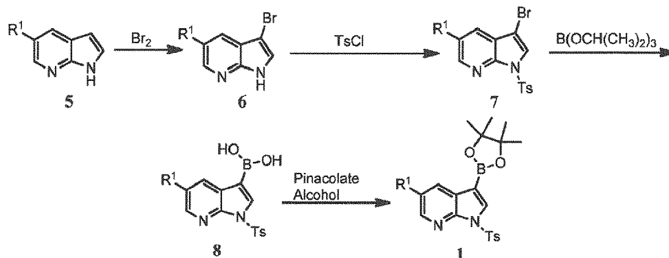
Scheme II:
