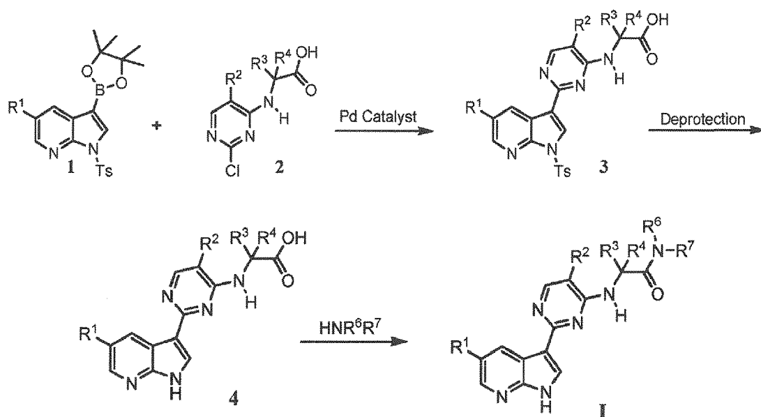
Scheme I:
