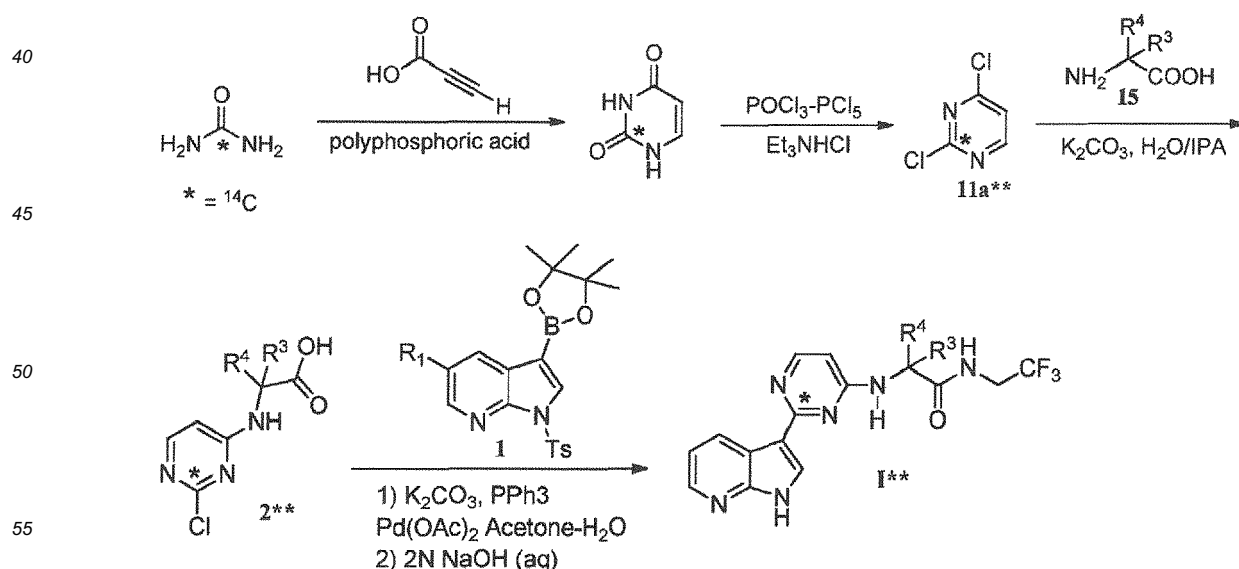
Scheme IV:
