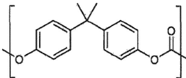
[Formule chimique 1-1]
