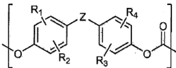
[Formule chimique 1]
