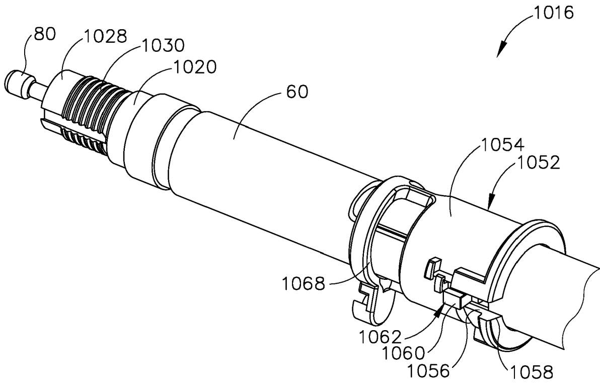
Fig.20A
