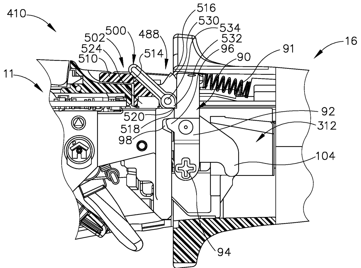
Fig.10A
