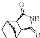
(3a R ,4 S ,7 R ,7a S )-hexahydro-1 H - 4,7-methanoisoindole-1,3(2 H )- dione
