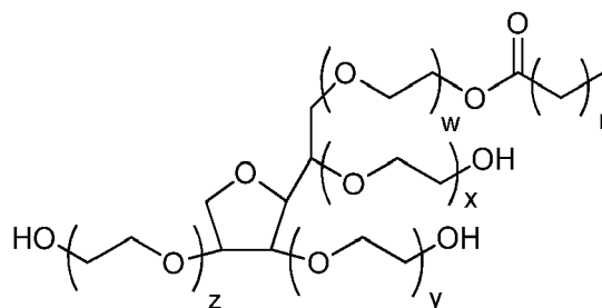
Polysorbate 20
