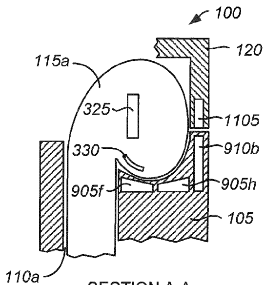
SECTION A-A FIG. 11
