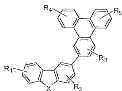
Compound 6G
