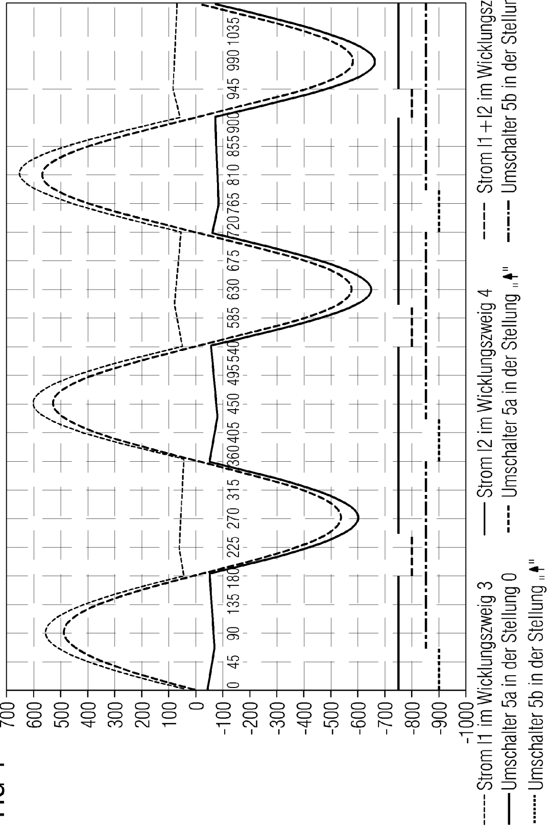
FIG 4 Ströme I1, I2, I1 + I2 in den Wicklungen 3, 4, A
