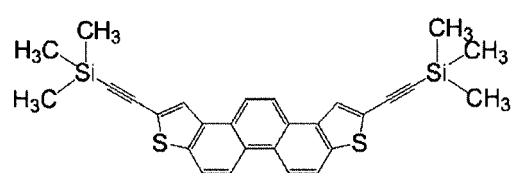
OSC-64
