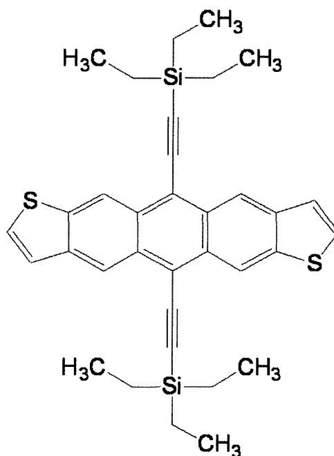
OSC - 18
