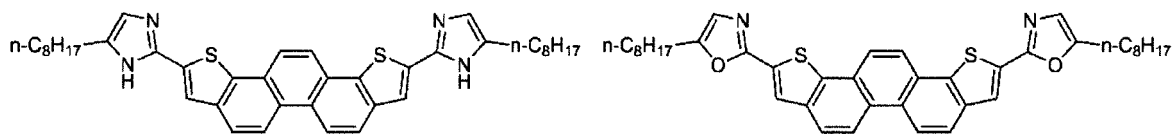
OSC-52
