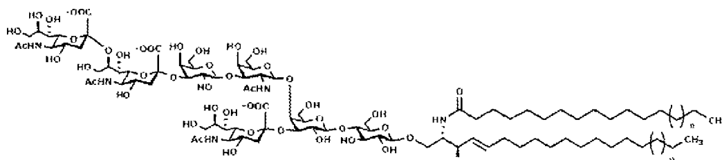
GT1a
