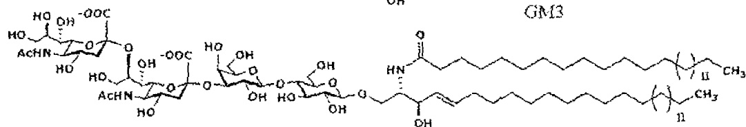
GD3
