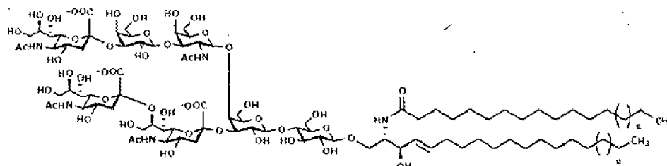
GT1b
