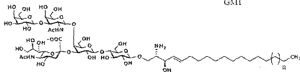
Lyso-GM1
