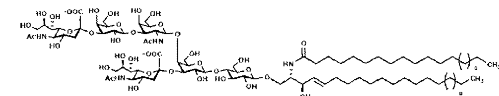
GD1a
