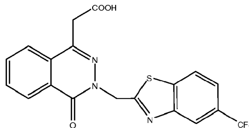
zopolrestat
