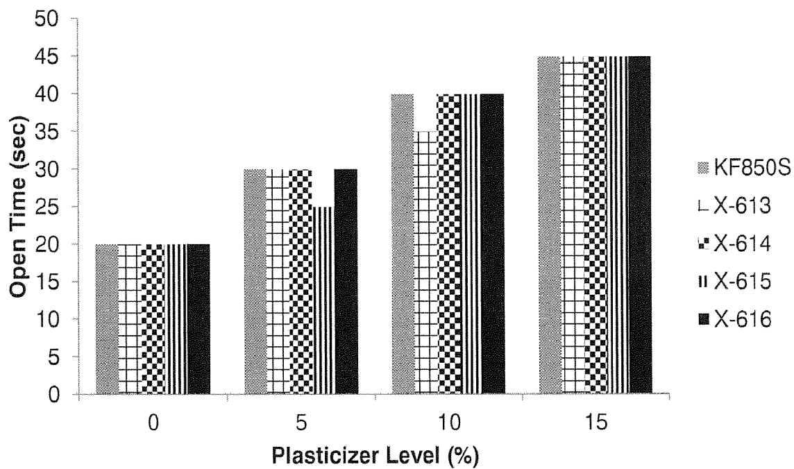
FIG. 29 -- Copolymer Open Times
