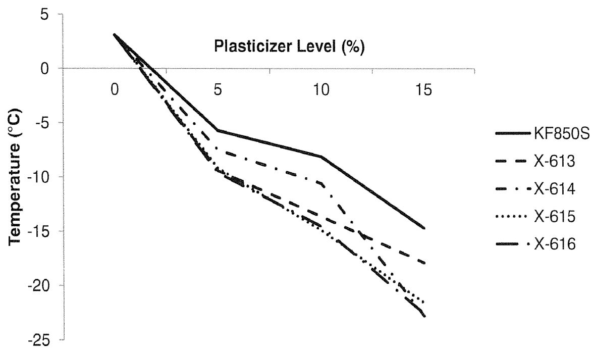
FIG. 27 -- Tg Suppression - Copolymer
