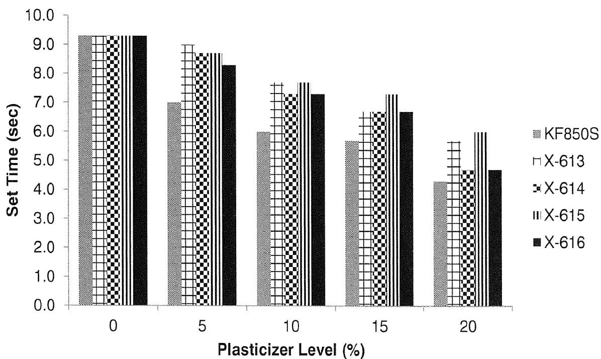
FIG. 35 -- Set Times - Homopolymer
