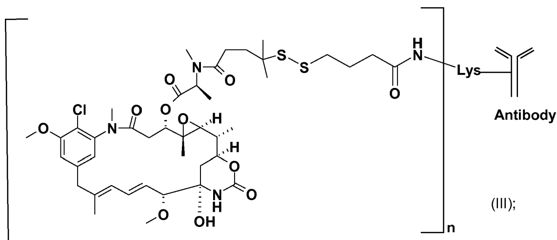
Ab-SPDB-DM4
